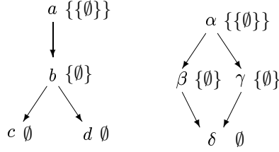
ΔΙΑΓΡΑΜΜΑ B.2. Μη ισομορφικά, προσόμοια, εδραιωμένα γραφήματα.
