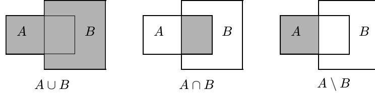
ΔΙΑΓΡΑΜΜΑ 1.1. Πράξεις Boole.
