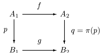
ΔΙΑΓΡΑΜΜΑ 1. Διάγραμμα για την Άσκηση 2.23.
