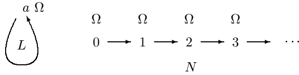
ΔΙΑΓΡΑΜΜΑ B.3. Πολλές εικόνες του \Omega : το (L, a) και κάθε (N, n) .
