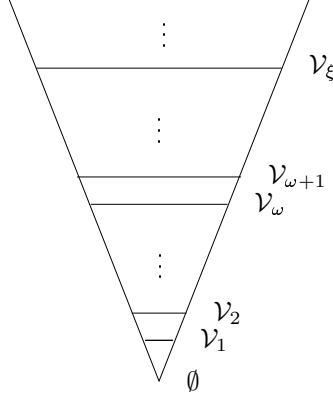
ΔΙΑΓΡΑΜΜΑ 12.3. Λογαριθμική απόδοση των αγνών, εδραιωμένων συνόλων.
